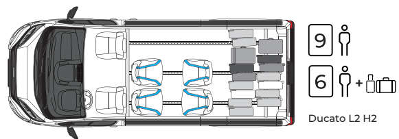
Esempio possibile configurazione Passo Medio. Example of a Medium Wheelbase configuration.
